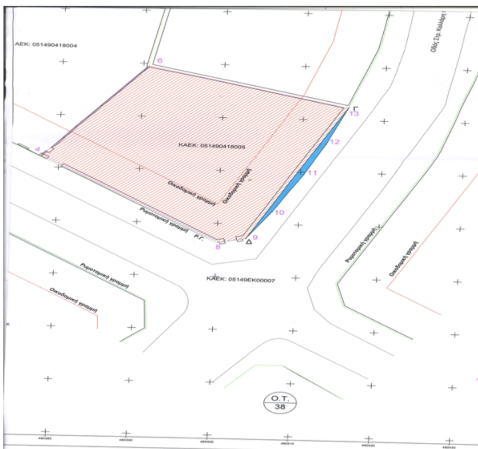
Εικόνα 1. Απόσπασμα τοπογραφικού διαγράμματος T-1 του Δημητρίου Α. Καπνιά, αγρ. τοπογράφου μηχανικού
