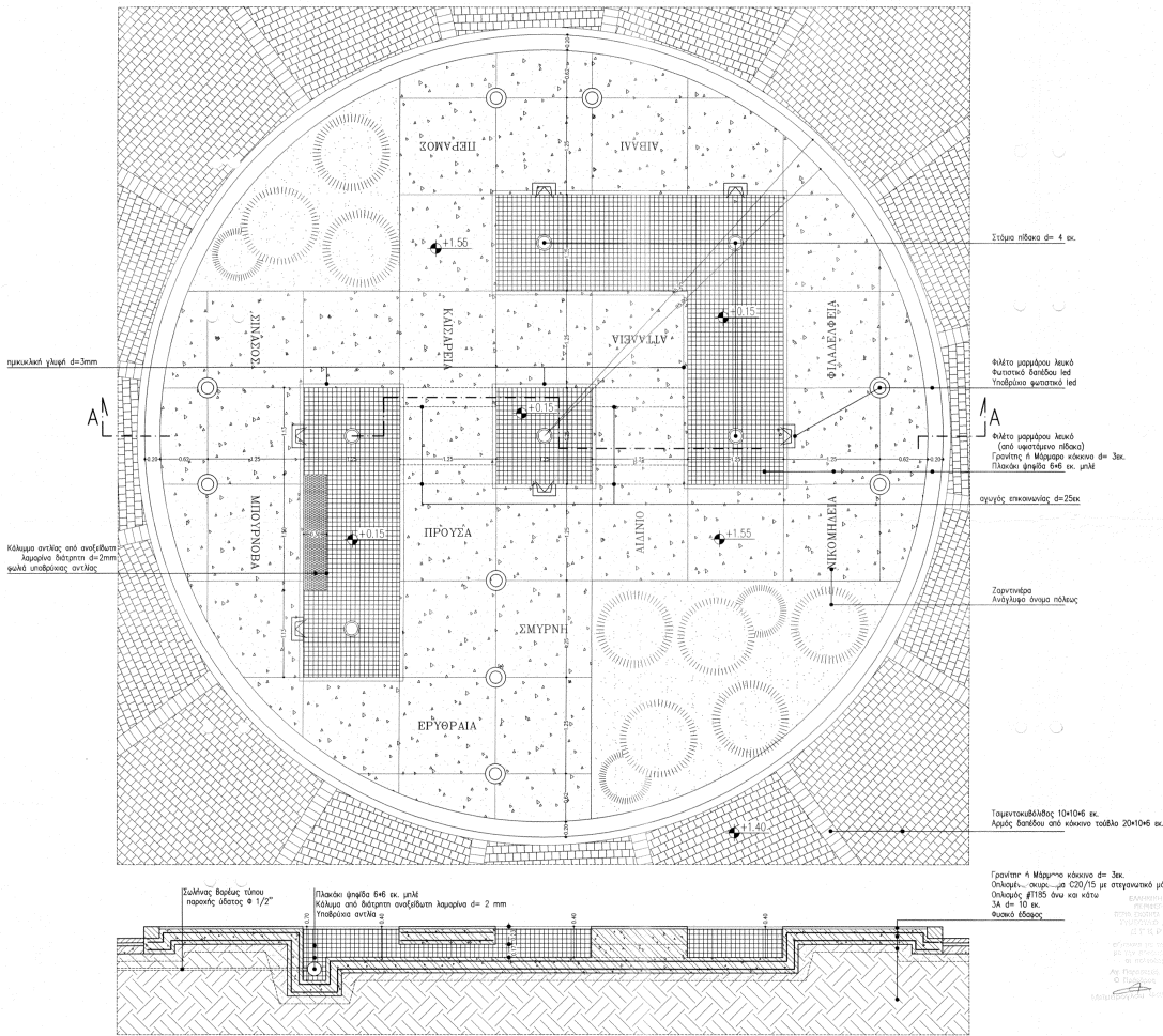
ΤΟΜΗ ΠΛΑΚΑ Κλίμακα: 1:25
