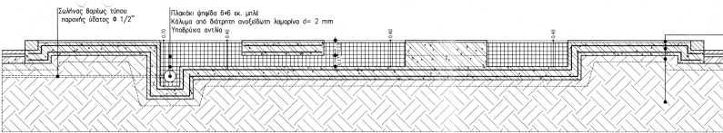
ΤΟΜΗ ΠΛΑΚΑ Κλίμακα: 1:25
