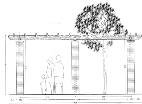
A24 ΠΡΟΣΩΠΗ Κλίμακα: 1:25
