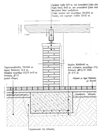
A25 ΤΟΜΗ Β - ΒΕΜΕΛΙΩΣΗ ΠΕΡΙΚΟΛΑΣ Κλίμακα: 1:10
