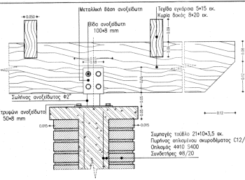
A26 ΤΟΜΗ Γ - ΛΕΠΤΟΜΕΡΙΑ ΣΤΗΡΙΞΗΣ ΠΕΡΙΚΟΛΑΣ Κλίμακα: 1:5
