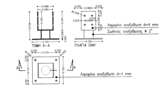
A27 ΜΕΤΑΛΛΙΚΗ ΒΑΣΗ ΠΕΡΙΚΟΛΑΣ ΑΝΟΣΩΒΩΤΗ Κλίμακα: 1:5
