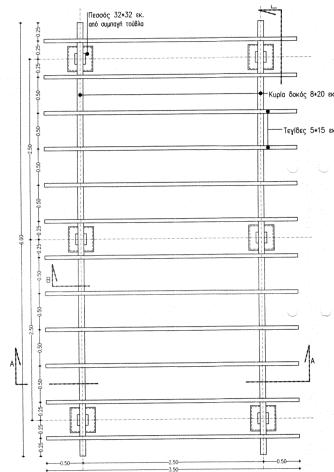
A21 ΚΑΤΩΗ ΣΤΗΡΙΞΗΣ ΠΕΡΙΚΟΛΑΣ Κλίμακα: 1:25
