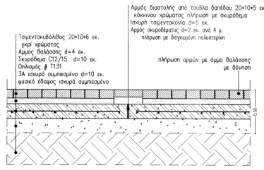
Α32 ΕΠΙΣΤΡΩΣΗ ΔΑΠΕΔΟΥ ΜΕ ΤΣΙΜΕΝΤΟΚΥΒΑΝΘΟΥΣ ΣΕ ΑΡΜΟ ΔΙΑΣΤΩΗΣ Κλίμακα: 1:10
