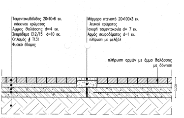
Α34 ΕΠΙΣΤΡΩΣΗ ΠΕΖΟΔΡΟΜΟΥ ΣΕ ΑΡΜΟ ΔΙΑΣΤΩΗΣ Κλίμακα: 1:10
