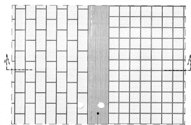
ΚΑΤΩΗ ΠΛΑΚΟΣΤΡΩΣΗ Απός διαστολής με μάρμαρο
