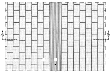
ΚΑΤΩΗ ΠΛΑΚΟΣΤΡΩΣΗ Απός πλακοστρώσης με μάρμαρο ανά 20 μ. max
