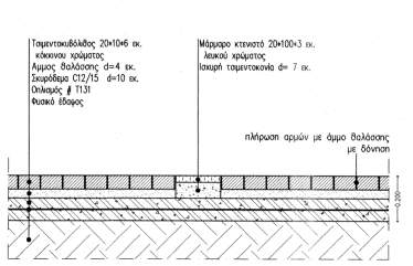
Α35 ΕΠΙΣΤΡΩΣΗ ΠΕΖΟΔΡΟΜΟΥ ΣΕ ΑΡΜΟ ΕΓΚΙΒΩΤΙΣΜΟΥ Κλίμακα: 1:10
