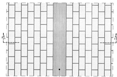
ΚΑΤΩΗ ΠΛΑΚΟΣΤΡΩΣΗ Απός εγκιβωτισμού με μάρμαρο ανά 3 μ. min
