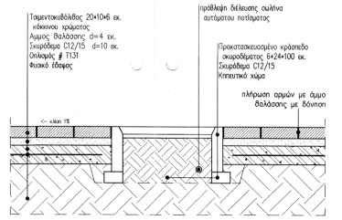
Α33 ΕΠΙΣΤΡΩΣΗ ΠΕΖΟΔΡΟΜΟΥ ΣΕ ΦΩΛΙΑ ΔΕΝΔΡΟΥ Κλίμακα: 1:10
