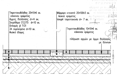
Α36 ΕΠΙΣΤΡΩΣΗ ΠΕΖΟΔΡΟΜΟΥ ΣΕ ΑΡΜΟ ΔΙΑΣΤΩΗΣ Κλίμακα: 1:10
