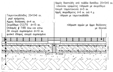
Α31 ΕΠΙΣΤΡΩΣΗ ΔΑΠΕΔΟΥ ΜΕ ΤΣΙΜΕΝΤΟΚΥΒΑΝΘΟΥΣ ΣΕ ΑΡΜΟ ΔΙΑΣΤΩΗΣ Κλίμακα: 1:10
