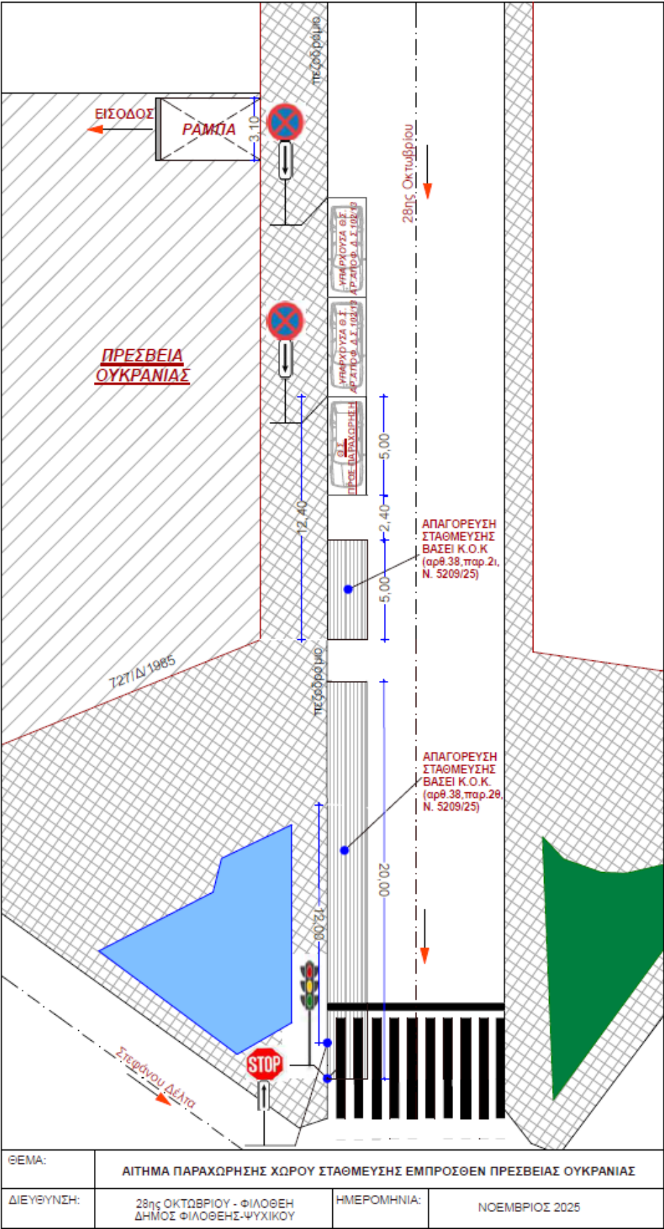
Σχεδιάγραμμα 1: Χωροθέτηση χώρου στάθμευσης προς παραχώρηση επί της οδού 28ης Οκτωβρίου, Φιλοθέη.
